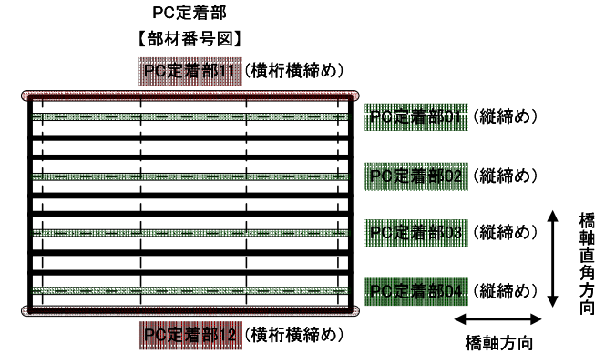
付図-9 PC 定着部の部材番号
