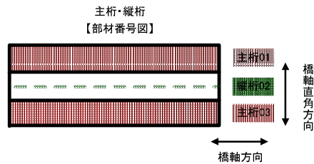
付図-3 箱桁橋等の部材番号
