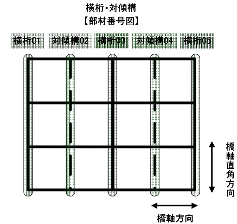
付図-5 横桁、対傾構の部材番号
