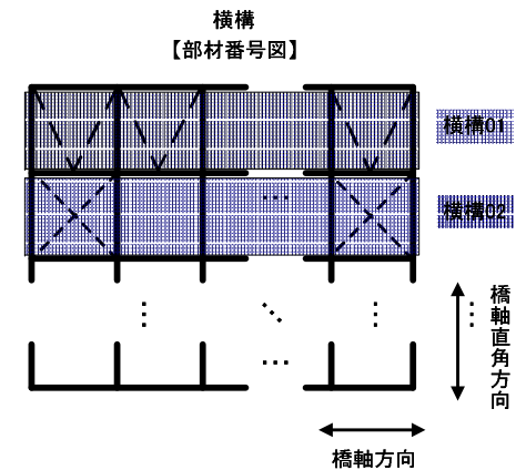
付図-6 横構の部材番号
