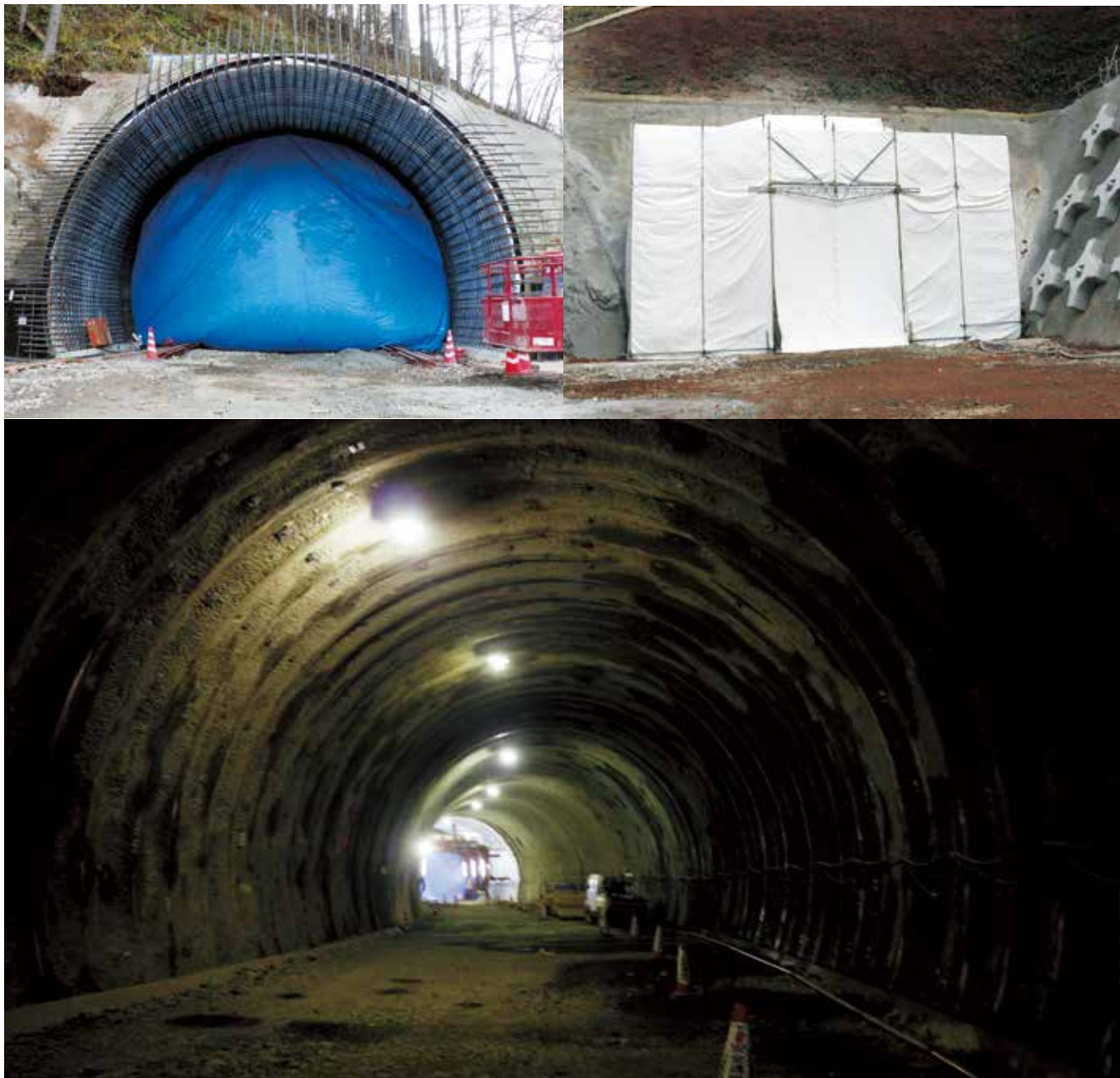
川上村大深山トンネル（2020/11/6）
